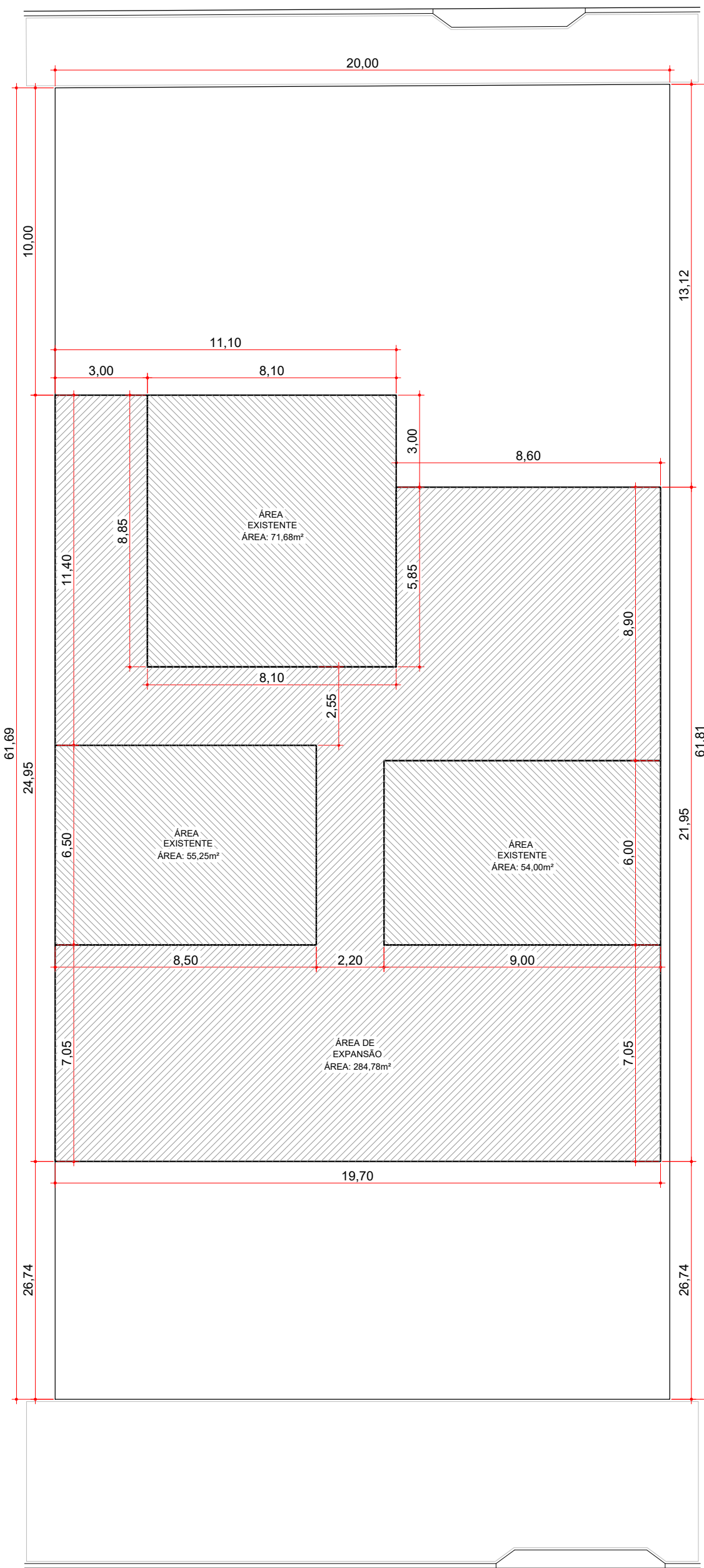
PLANILHA DE ÁREA ESCALA 1:200
