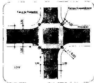
DETALHE GENÉRICO CRUZAMENTO VIAS 90° ESCALA 1:500
