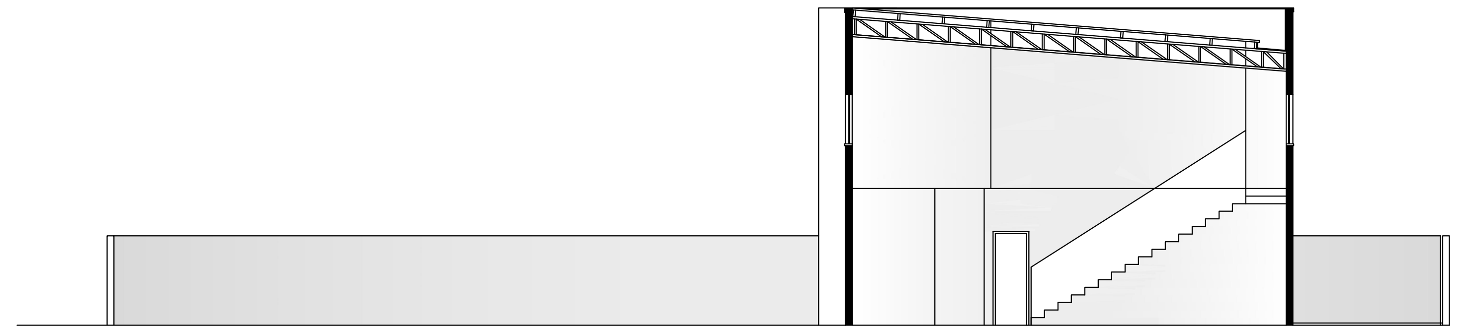
5 CORTE BB
