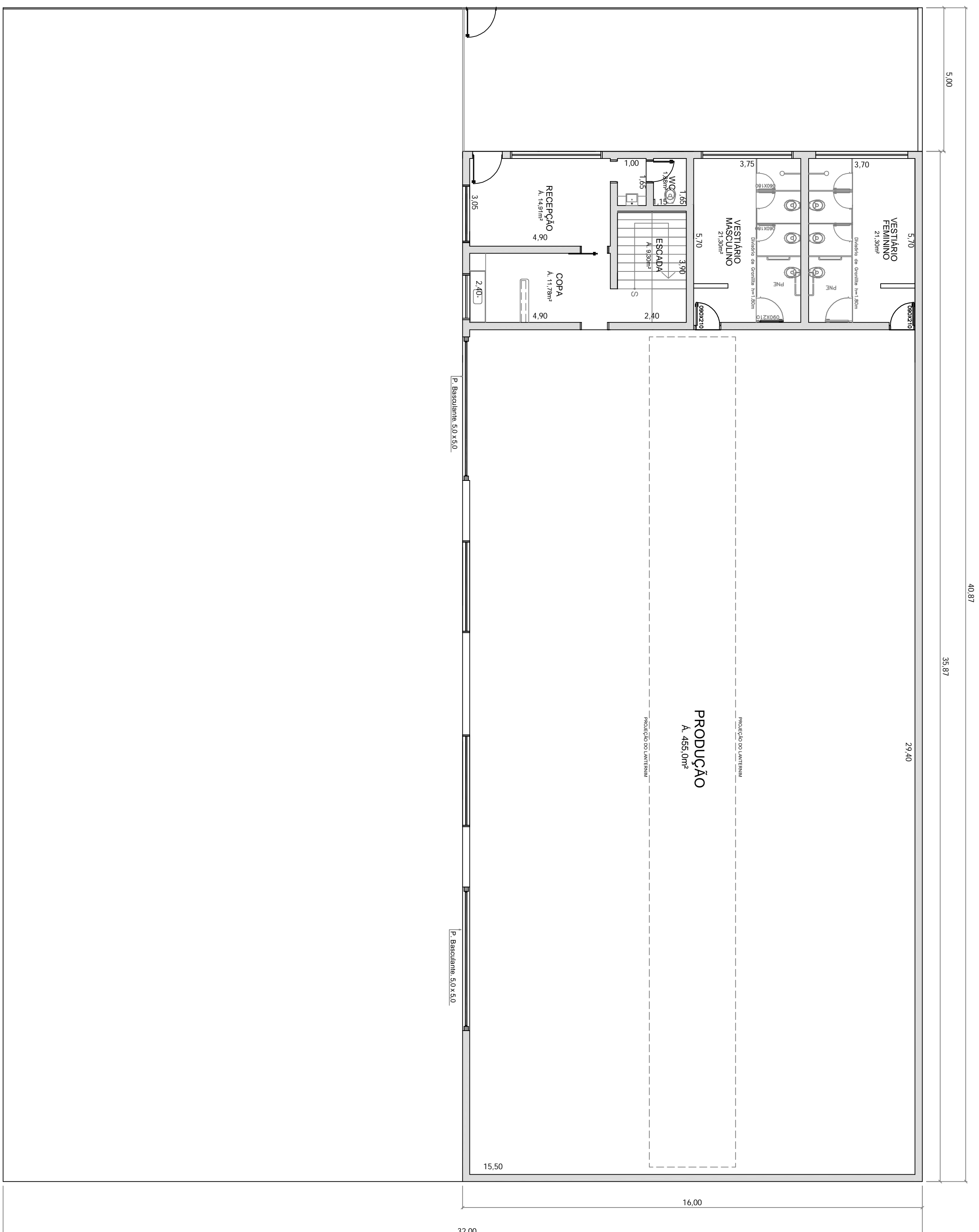
PLANTA TÉCNICA ESC. 1:100
