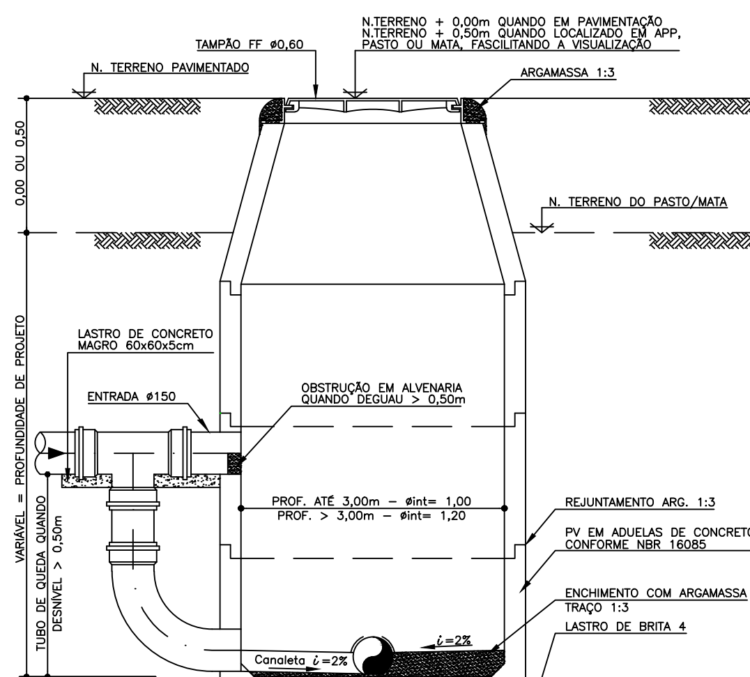
DET. DO POÇO DE VISITA ESC. 1:20 (Medidas em metros)
